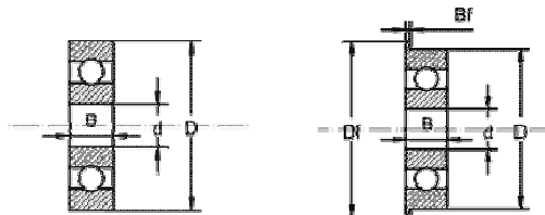
Kogellagers U en UF
