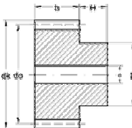
Tandwiel met Naaf (20 of 45 gr.)
